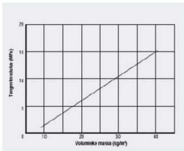
Figure 24: Relatie tangentmodulus/volumieke massa.
