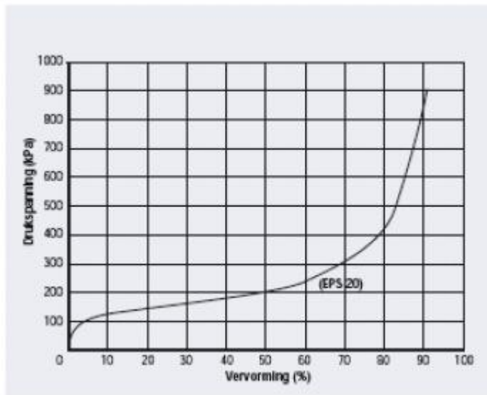
Figure 1: Last-vervormingsdiagram.
